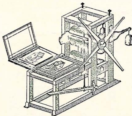
Eerste handpers (eigenlijk een plaatdrukker) door Senefelder gebruikt om proeven met steendruk te nemen. Tussen twee houten walsen werden steen en papier onder zware drukspanning doorgedraaid. Dit resulteerde spoedig in een gespleten bovenwals, zodat deze pers onbruikbaar werd.
