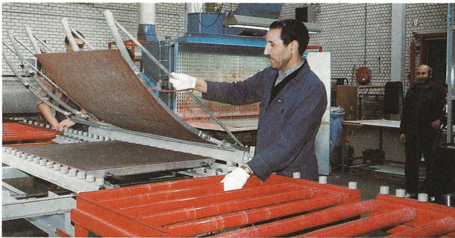
De gelijmde kunststof plaat wordt op de positioneertafel gelegd. Op deze tafel wordt de kunststof plaat precies op het reeds voorverwarmde blad gelegd.
